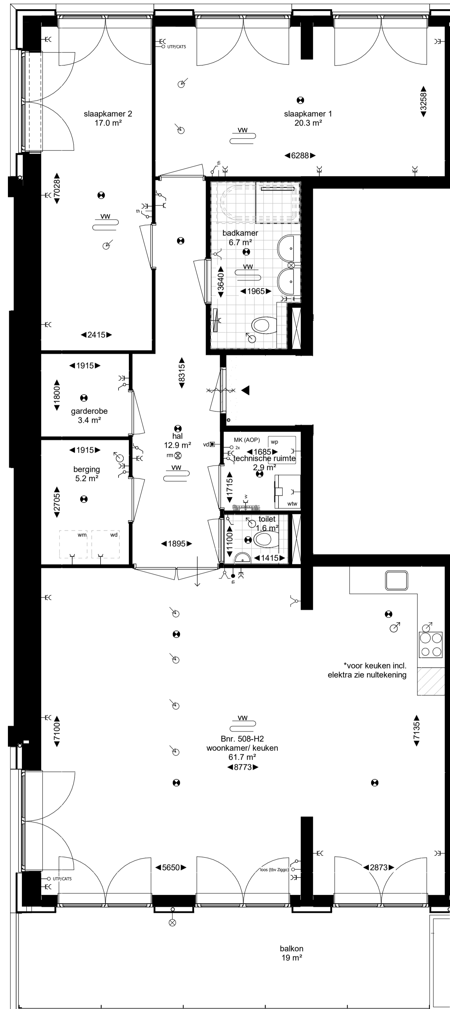
2e verdieping Maten in millimeters. Maten zijn 'circa' maten.
