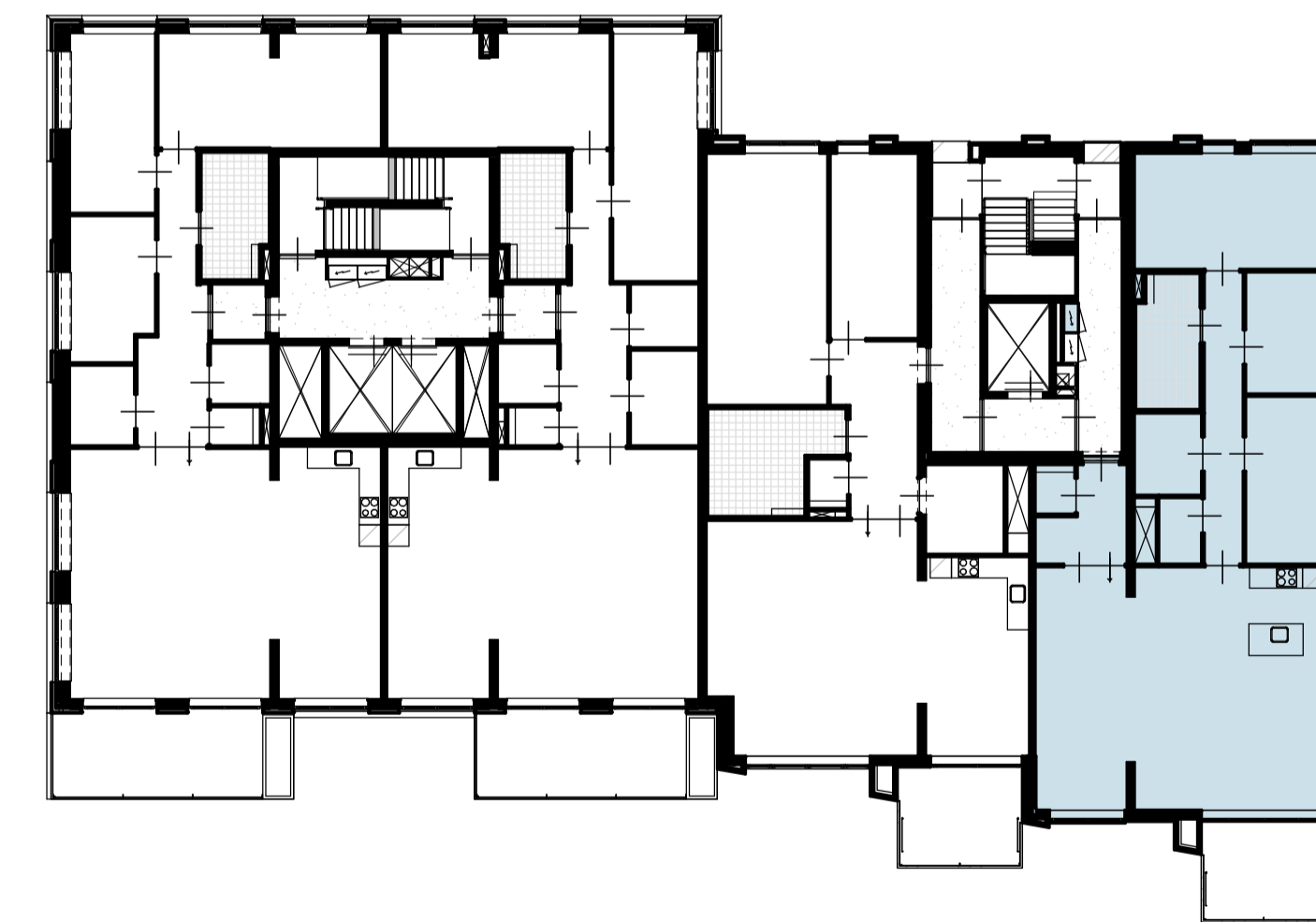
5e verdieping
