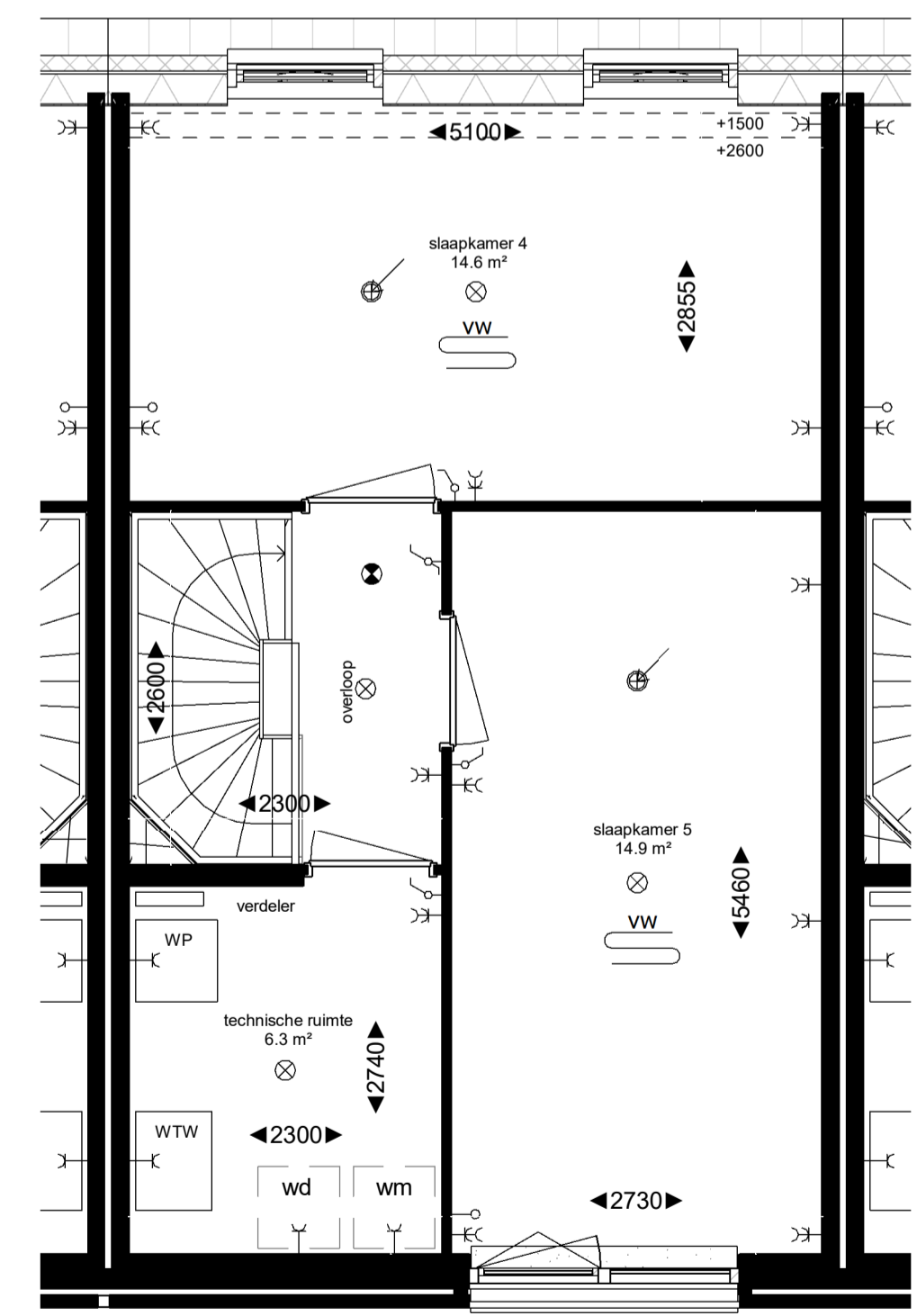
2e verdieping
