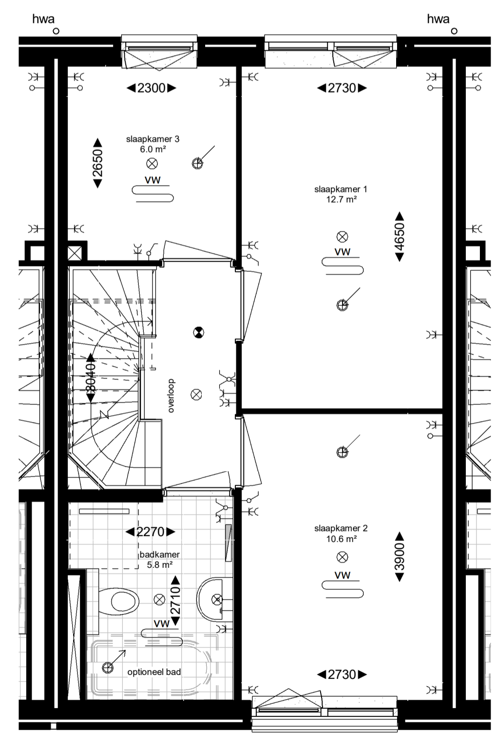
1e verdieping
