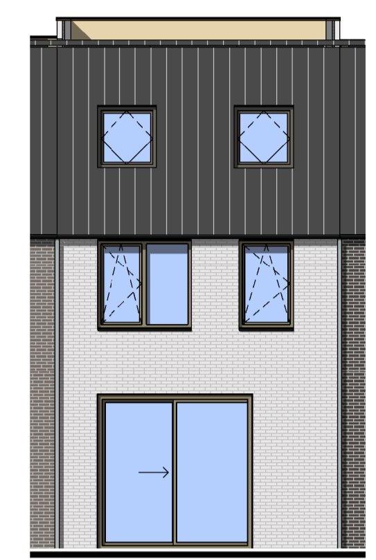
achtergevel (1:100)
