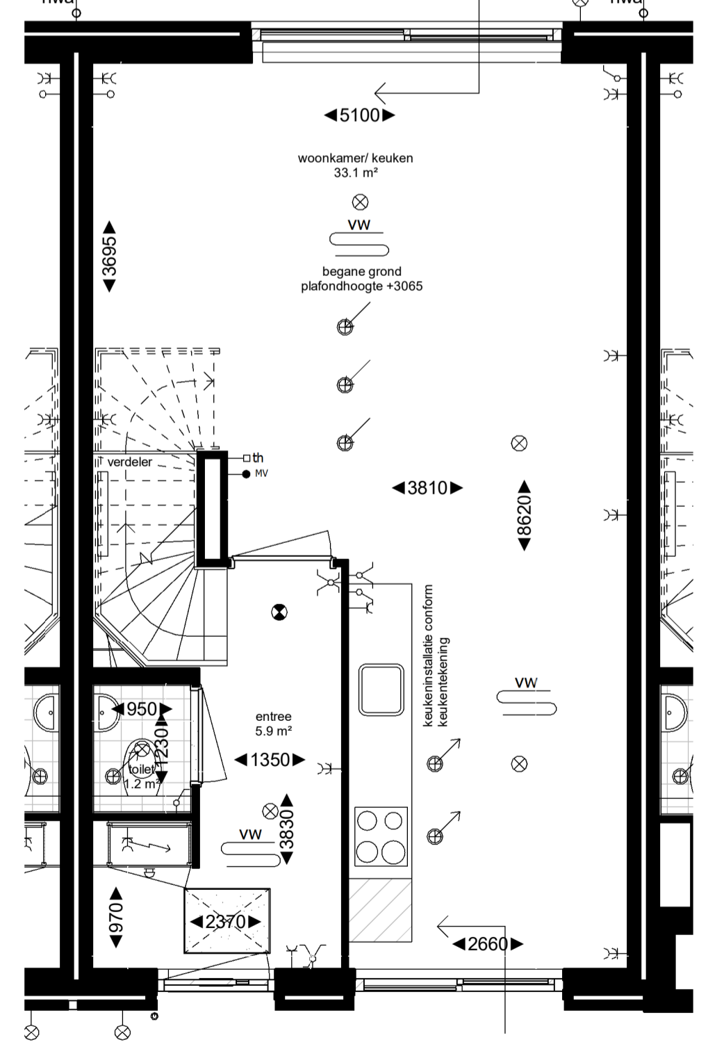
begane grond
