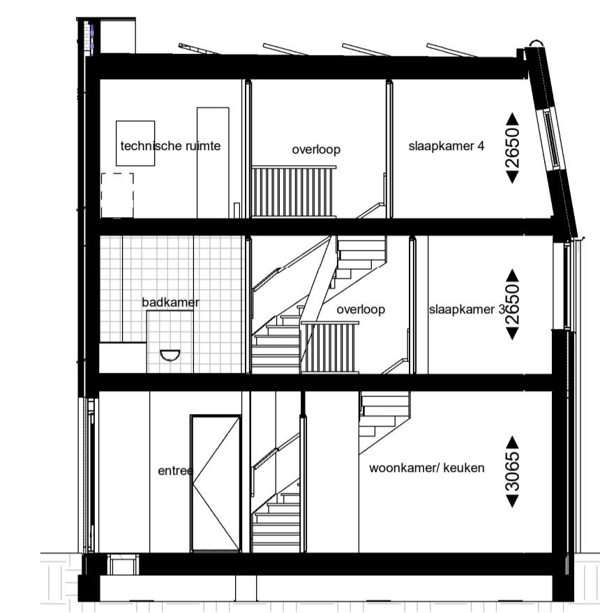
doorsnede (1:100)
