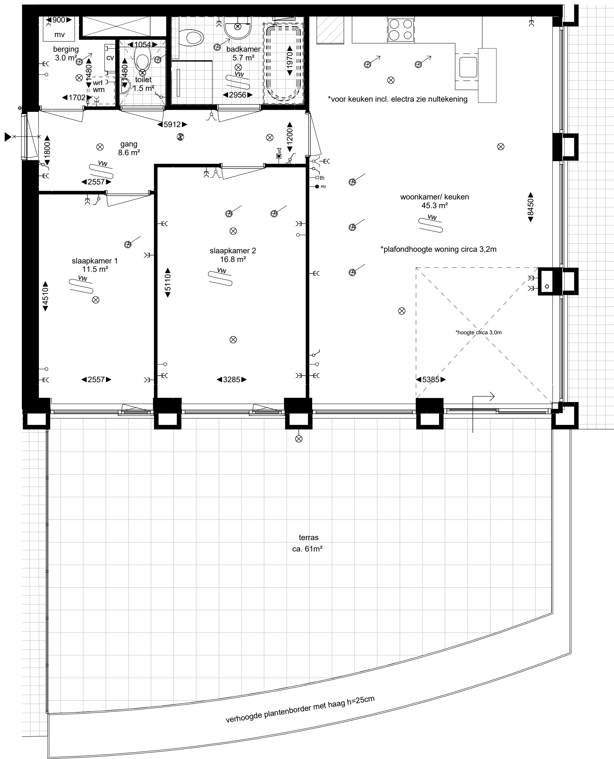
begane grond 1:50
