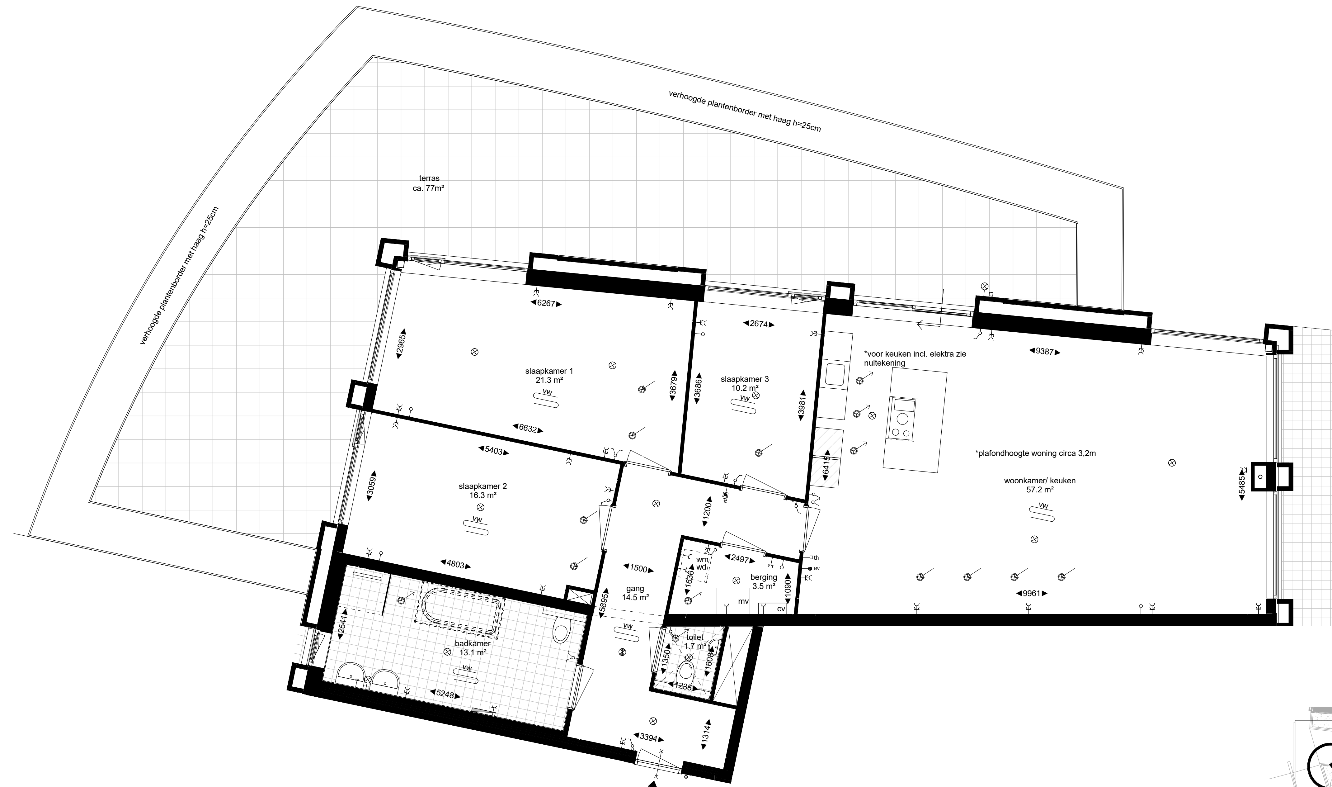
begane grond 1:50 Maten in mm. Maten zijn 'circa' maten
